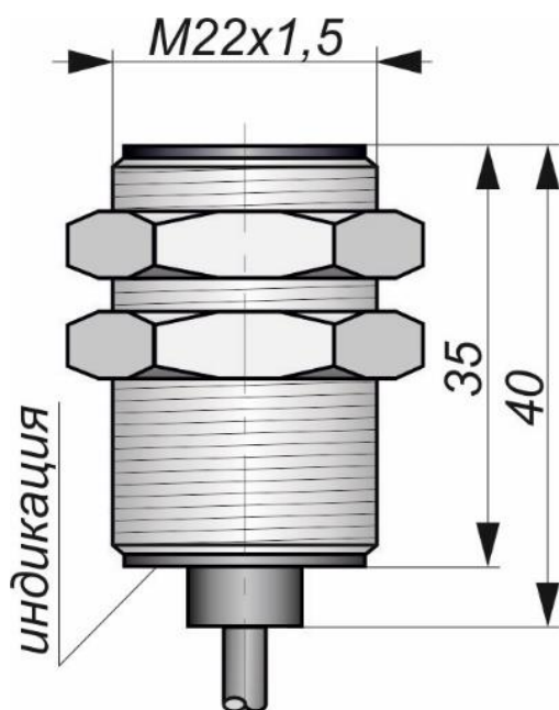
Габаритный чертеж
